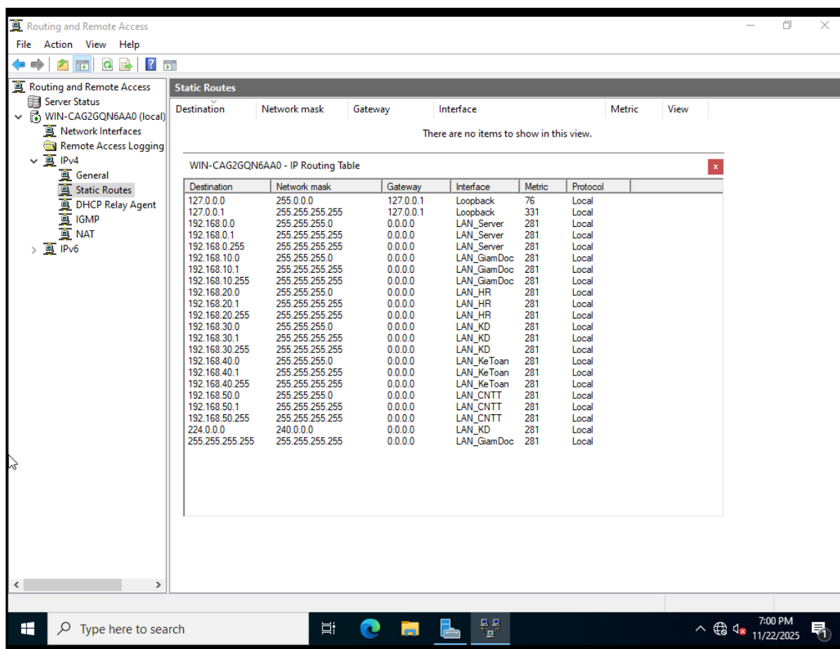
Hình 22: Bảng định tuyến hiển thị đầy đủ các đường đi đến các mạng con
